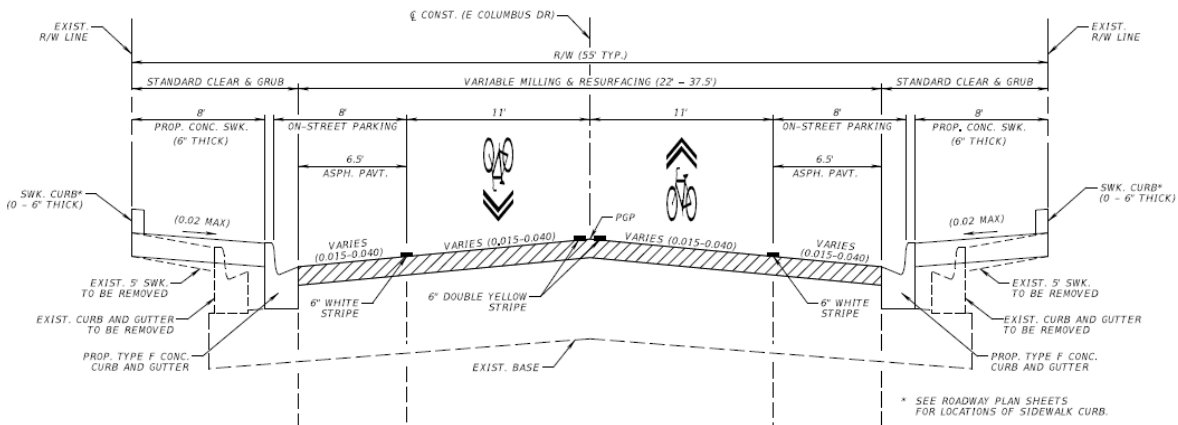
TYPICAL SECTION (N.T.S.) E COLUMBUS DR STA. 99+85.40 TO STA. 103+60.00 STA. 105+29.67 TO STA. 114+10.35 STA. 116+26.35 TO STA. 124+71.77
